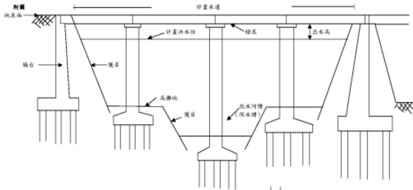
跨河建築物示意圖
